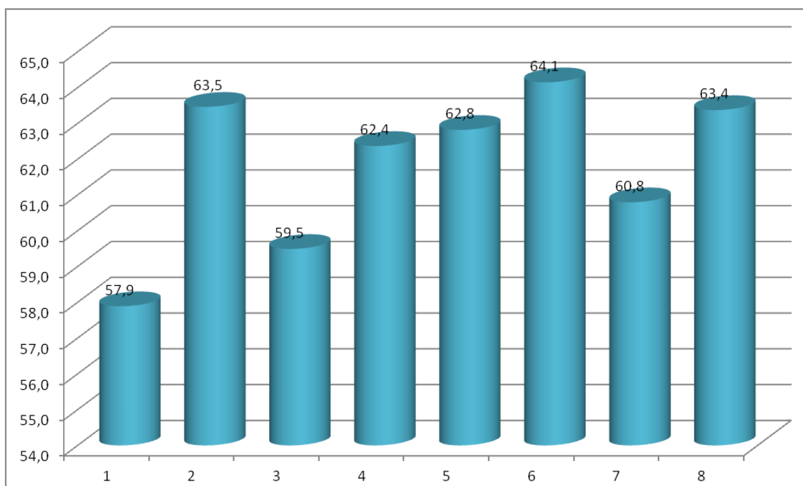
40 pav. Dienos, vakaro ir nakties triukšmo rodiklio ( L_{dvn} ) pasiskirstymas matavimo vietose. Ribinis dydis 65 dBA.
