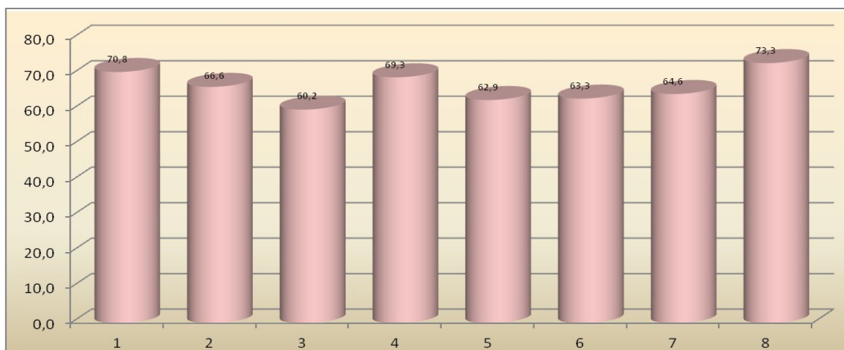
36 pav. Maksimalaus triukšmo pasiskirstymas matavimo vietose vakaro metu (18-22val.). Ribinis dydis 65 dBA.
