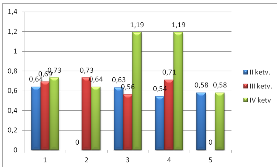
7 pav. Benzeno koncentracijų pasiskirstymas 2013 metais.
