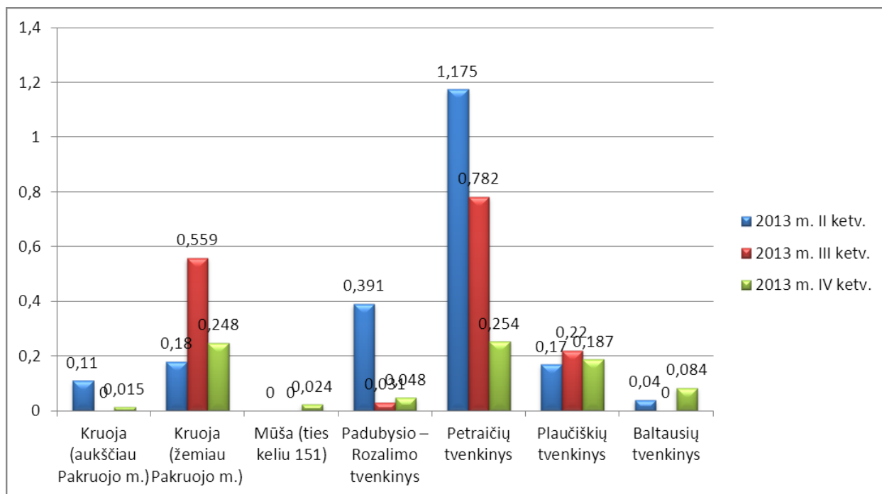
18 pav. \text{NH}_4\text{-N} koncentracija Pakruojis rajono paviršiniuose vandens telkiniuose.
