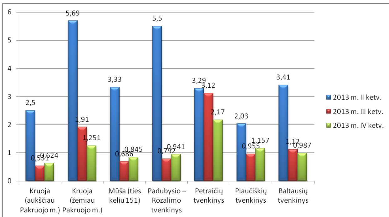
20 pav. N_b koncentracija Pakruojų rajono paviršiniuose vandens telkiniuose.
