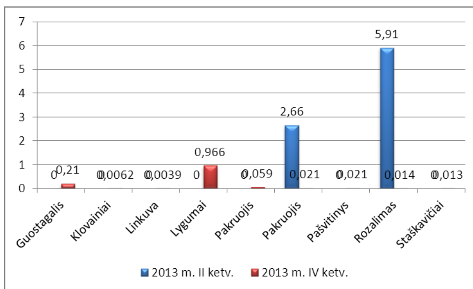
30 pav. Nitritų koncentracija Pakruojų rajono požeminiame vandenyje
