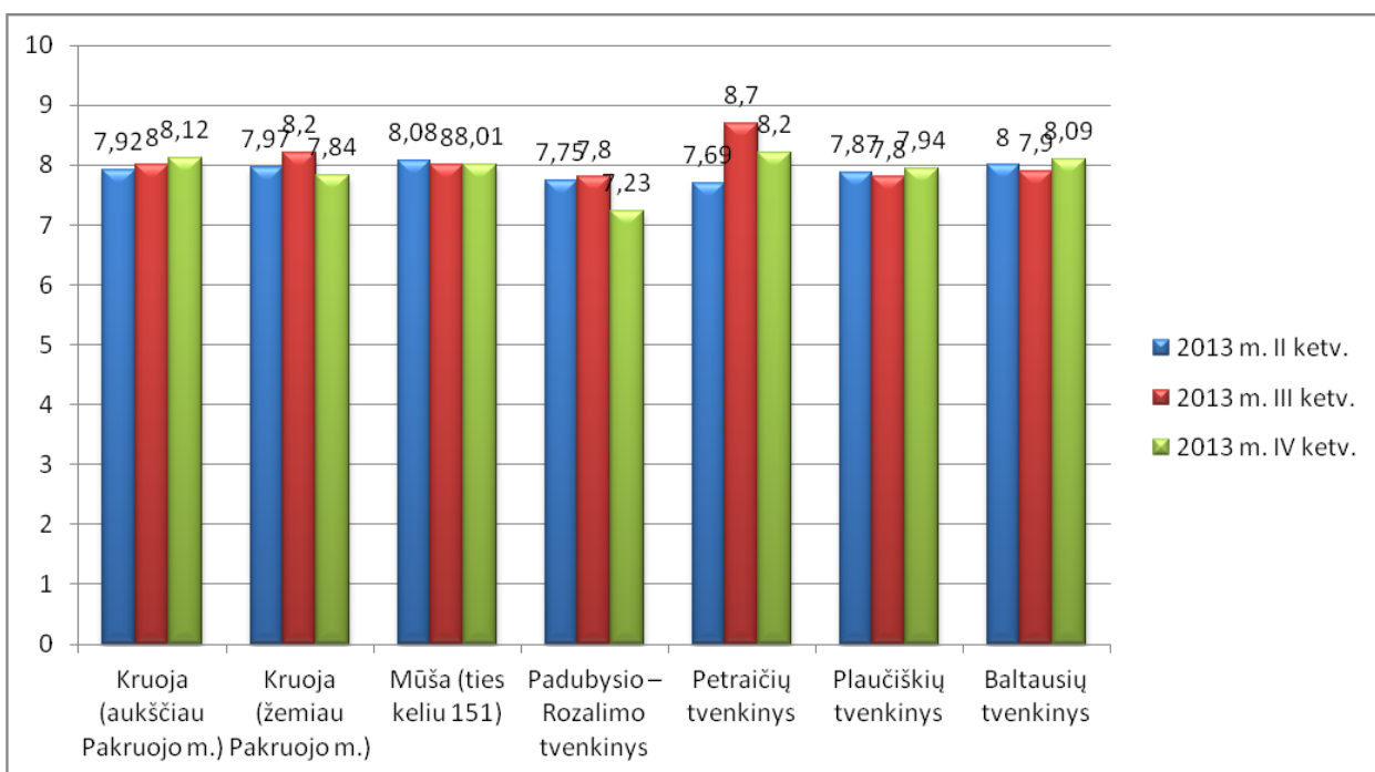
13 pav. pH vienetų skaičius Pakruojos rajono paviršiniuose vandens telkiniuose.
