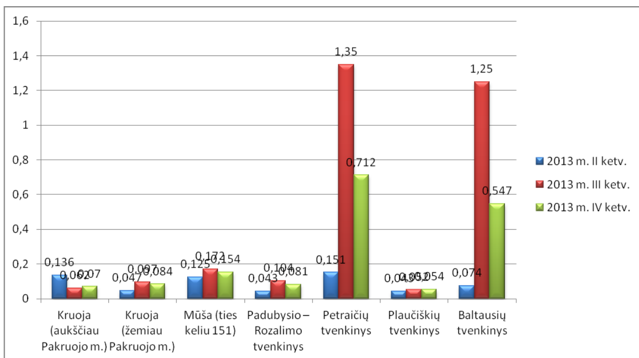
21 pav. P_b koncentracija Pakruojų rajono paviršiniuose vandens telkiniuose.
