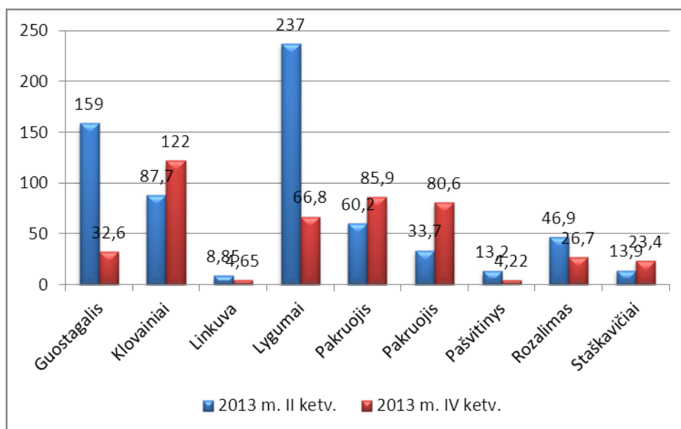
28 pav. nitratų koncentracija Pakruojo rajono požeminiame vandenyje
