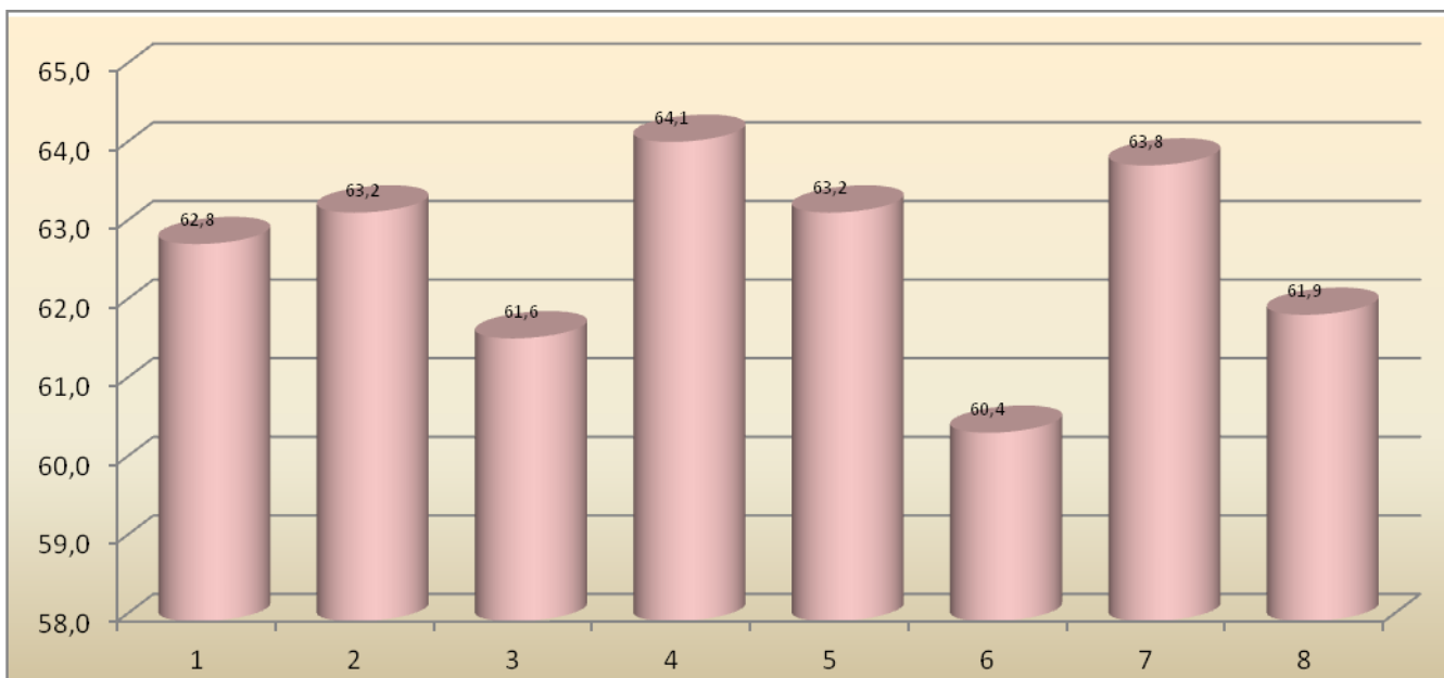
44 pav. Maksimalaus triukšmo pasiskirstymas matavimo vietose vakaro metu (18-22val.). Ribinis dydis 65 dBA.
