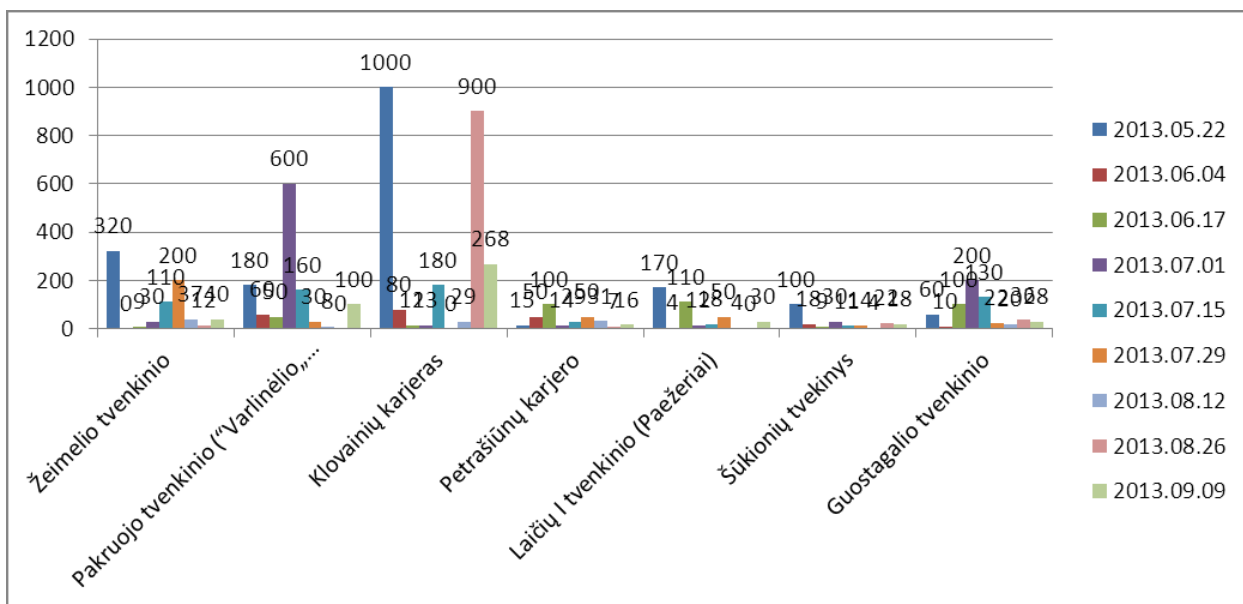
24 pav. E. Coli skaičius 100 ml. Pakruojos rajono maudykloje ir maudimvietėse
