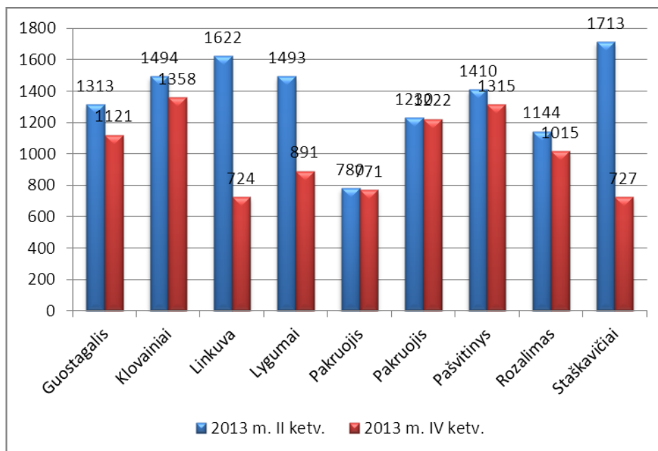
27 pav. Savitojo elektros laidžio koncentracija Pakruojo rajono požeminiame vandenyje
