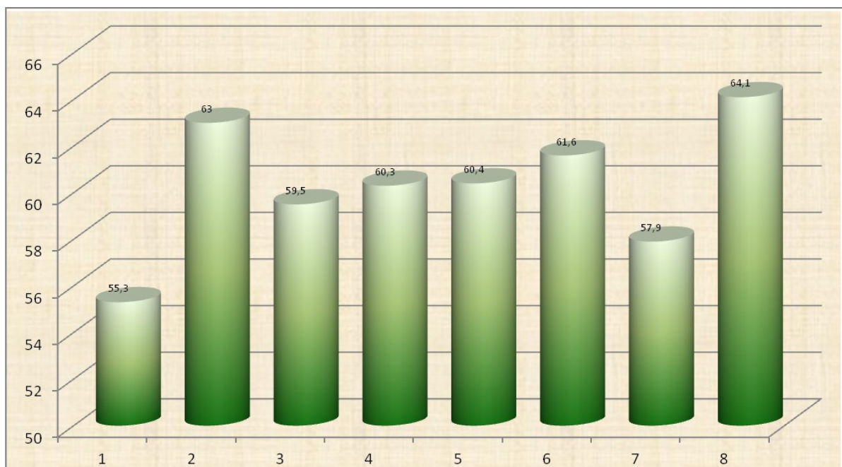
35 pav. Ekvivalentinio triukšmo pasiskirstymas matavimo vietose dienos metu (6-18 val.). Ribinis dydis 65 dBA.
