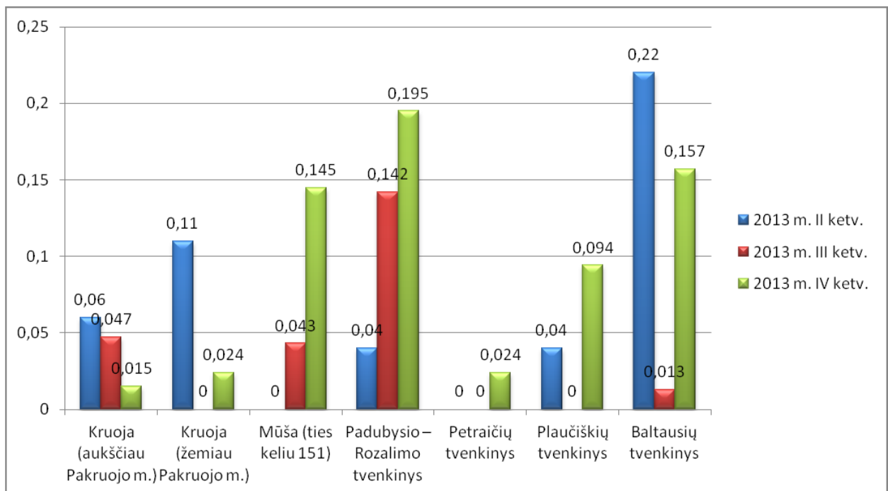
17 pav. NO 2 -N koncentracija Pakruojis rajono paviršiniuose vandens telkiniuose.
