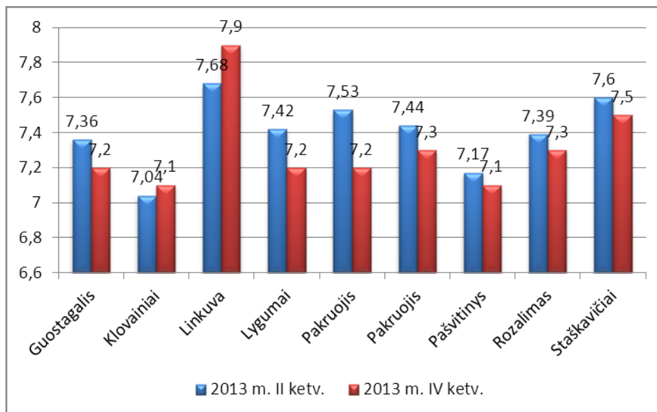
26 pav. pH koncentracija Pakruojo rajono požeminiame vandenyje
