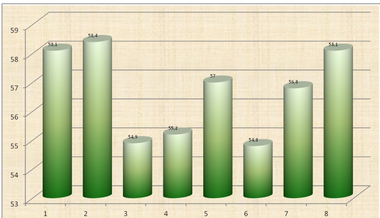
45 pav. Ekvivalentinio triukšmo pasiskirstymas matavimo vietose vakaro metu (18-22 val.). Ribinis dydis 60 dBA.
