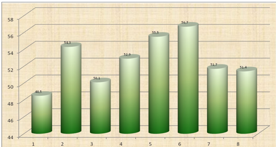
39 pav. Ekvivalentinio triukšmo pasiskirstymas matavimo vietose nakties metu (22-6 val.). Ribinis dydis 55 dBA.
