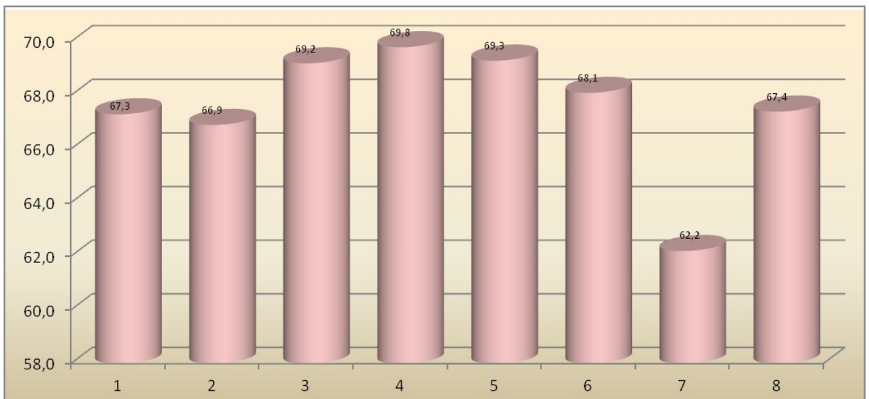
42 pav. Maksimalaus triukšmo pasiskirstymas matavimo vietose dienos metu (6-18 val.). Ribinis dydis 70 dBA.
