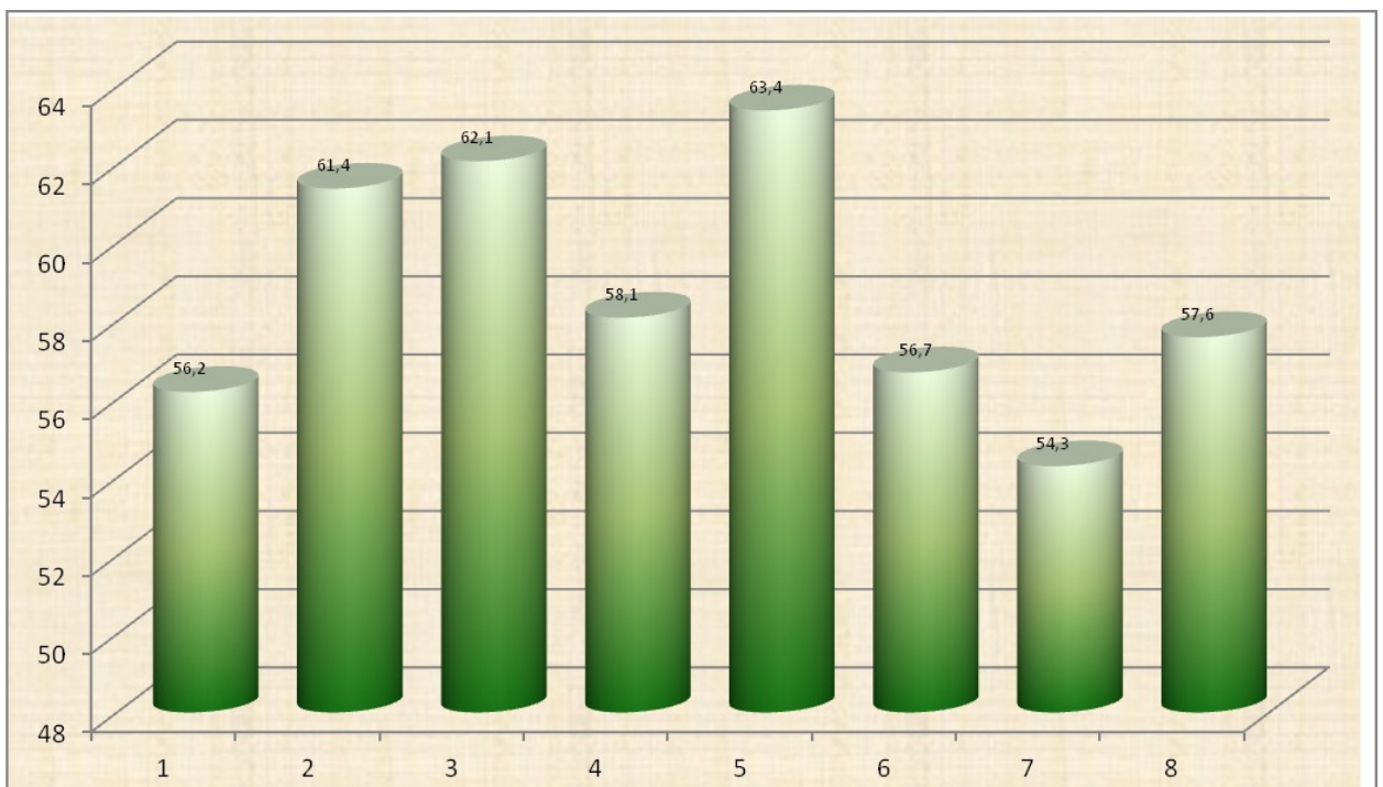
43 pav. Ekvivalentinio triukšmo pasiskirstymas matavimo vietose dienos metu (6-18 val.). Ribinis dydis 65 dBA.
