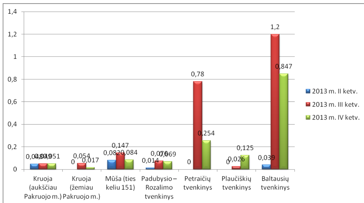
19 pav. \text{PO}_4\text{-P} koncentracija Pakruojis rajono paviršiniuose vandens telkiniuose.
