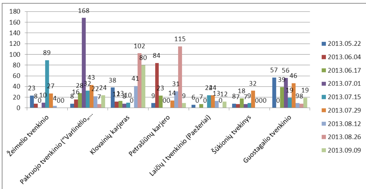
23 pav. Žarninių enterokokų skaičius 100 ml. Pakruojos rajono maudykloje ir maudimvietėse
