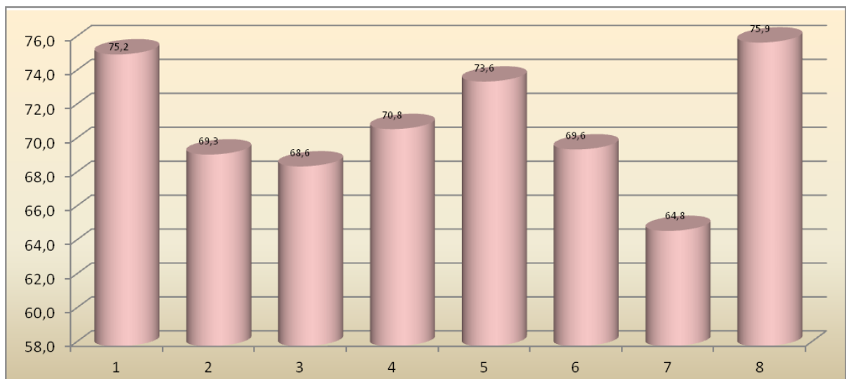
34 pav. Maksimalaus triukšmo pasiskirstymas matavimo vietose dienos metu (6-18val.). Ribinis dydis 70 dBA.
