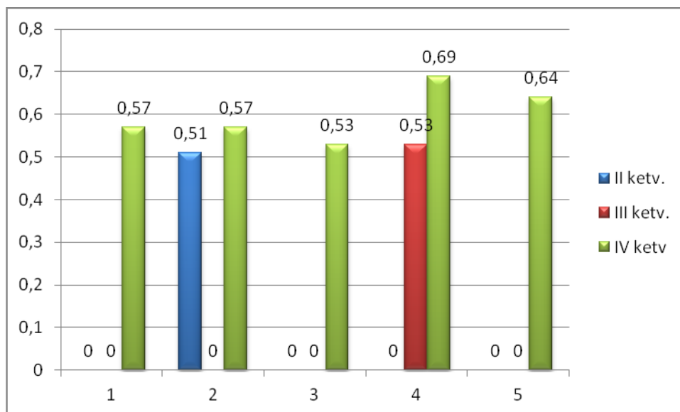
11 pav. O-ksileno koncentracijų pasiskirstymas 2013 metais.
