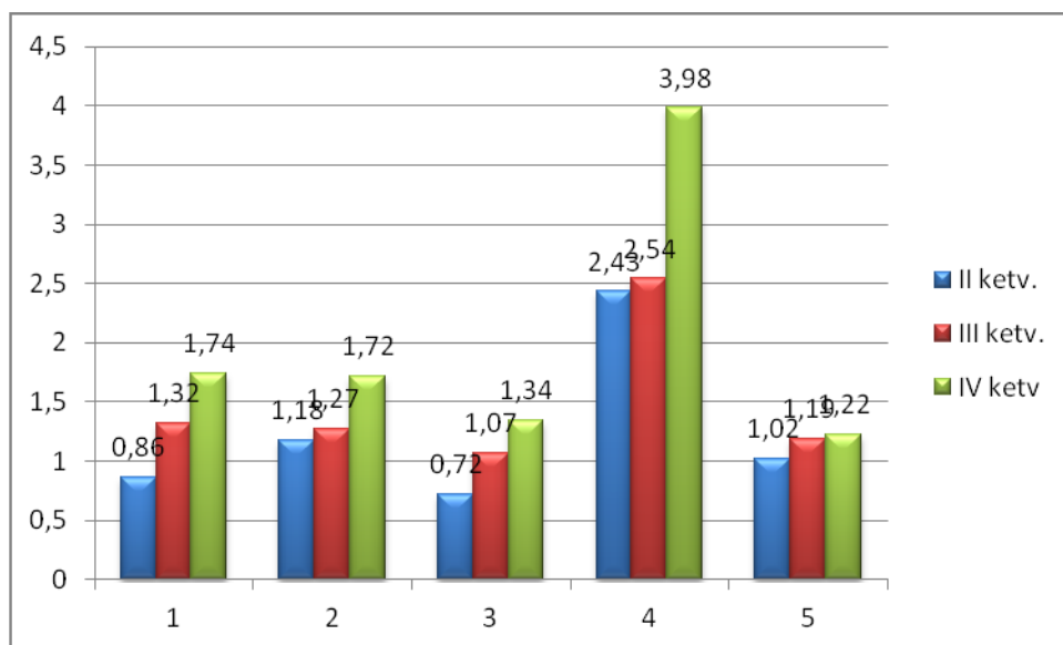
8 pav. Tolueno koncentracijų pasiskirstymas 2013 metais.
