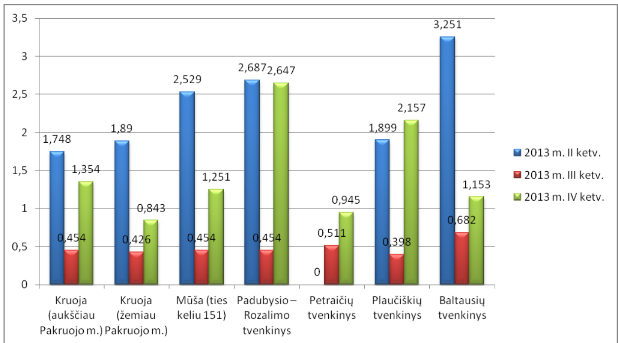
16 pav. NO 3 -N koncentracija Pakruojis rajono paviršiniuose vandens telkiniuose.
