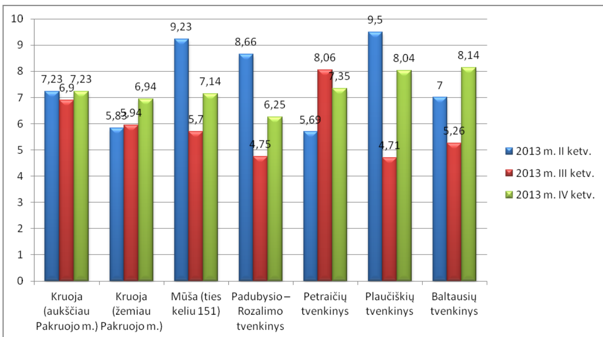
12 pav. O 2 koncentracija Pakruojos rajono paviršiniuose vandens telkiniuose.
