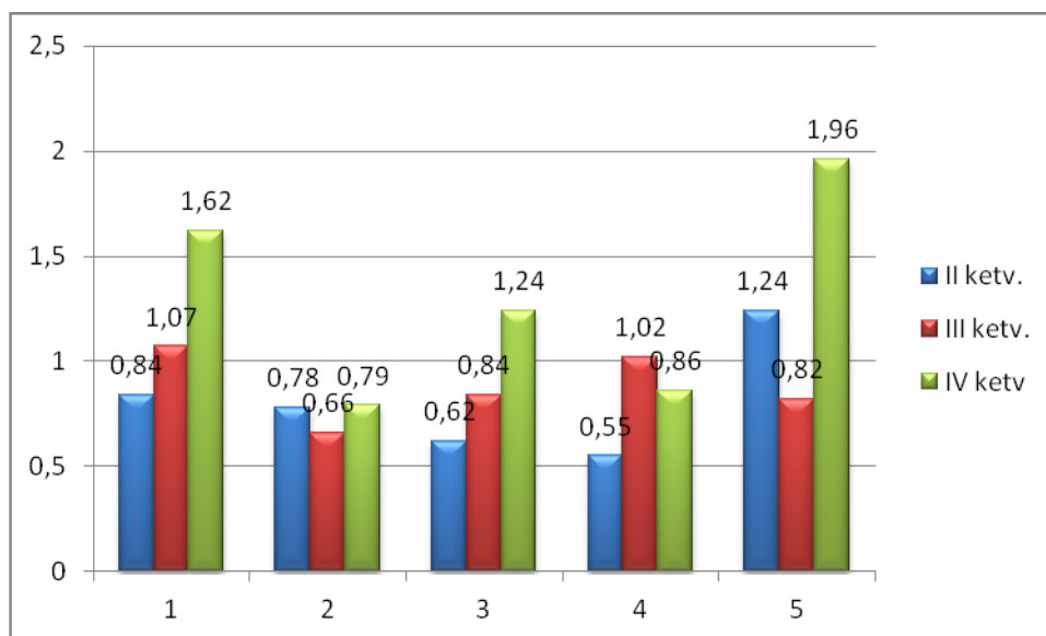
10 pav. M/p-ksileno koncentracijų pasiskirstymas 2013 metais.
