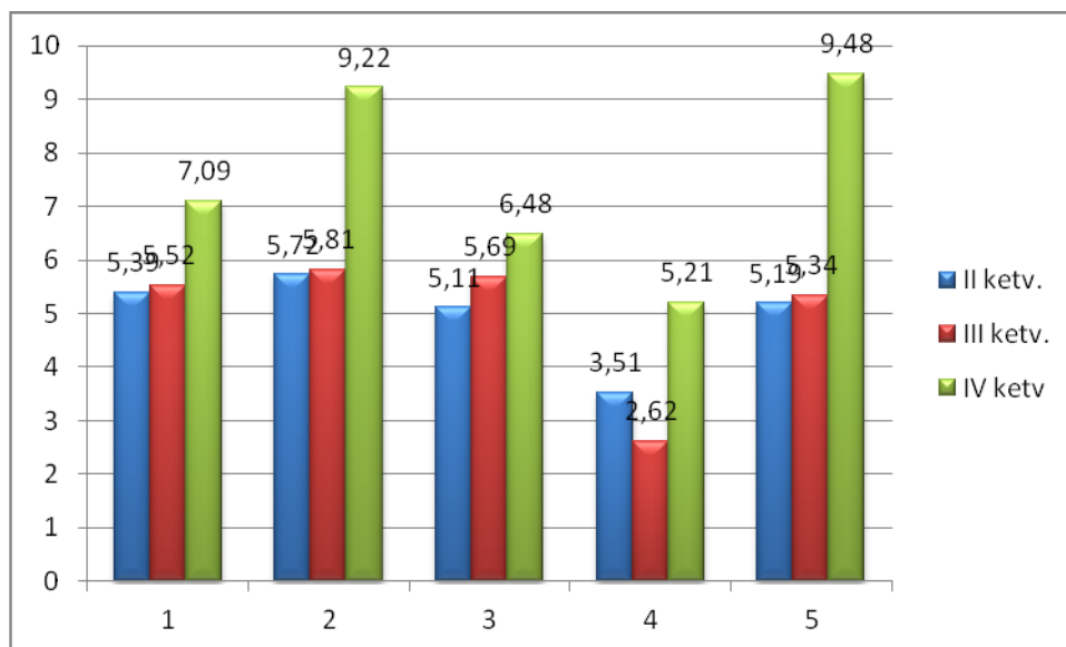
5 pav. NO 2 koncentracijų pasiskirstymas 2013 metais.
