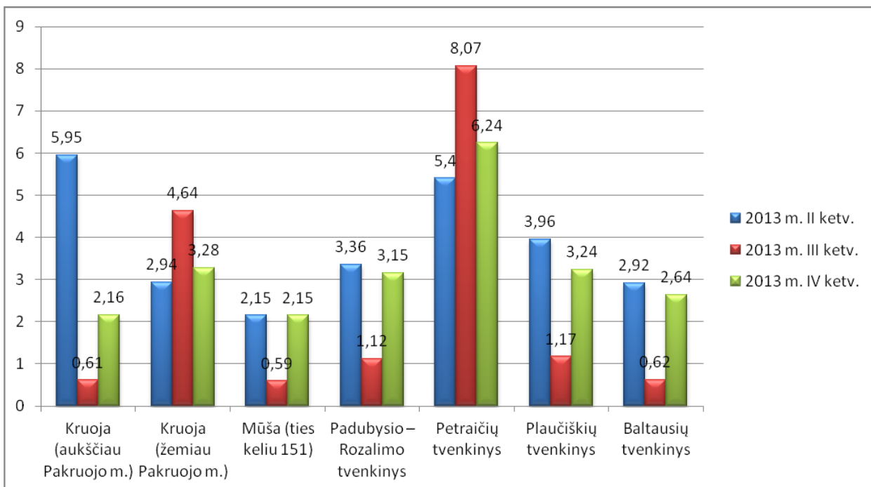
15 pav. BDS 7 koncentracija Pakruojos rajono paviršiniuose vandens telkiniuose.
