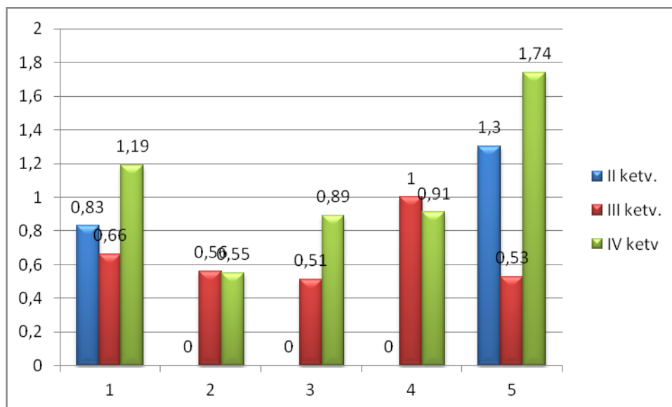
9 pav. Etilbenzeno koncentracijų pasiskirstymas 2013 metais.
