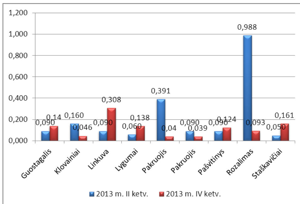
29 pav. Amonio azoto koncentracija Pakruojų rajono požeminiame vandenyje
