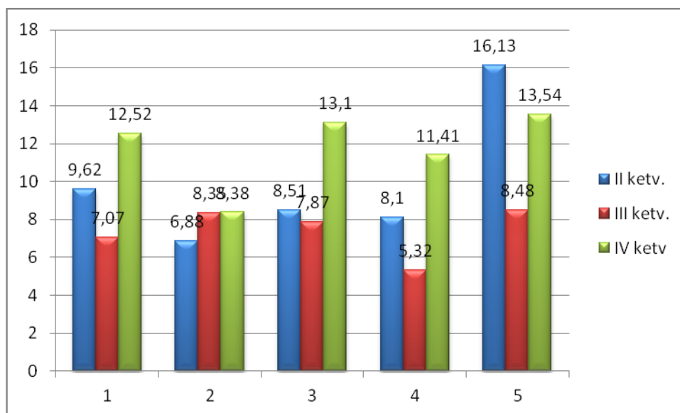
6 pav. SO 2 koncentracijų pasiskirstymas 2013 metais.
