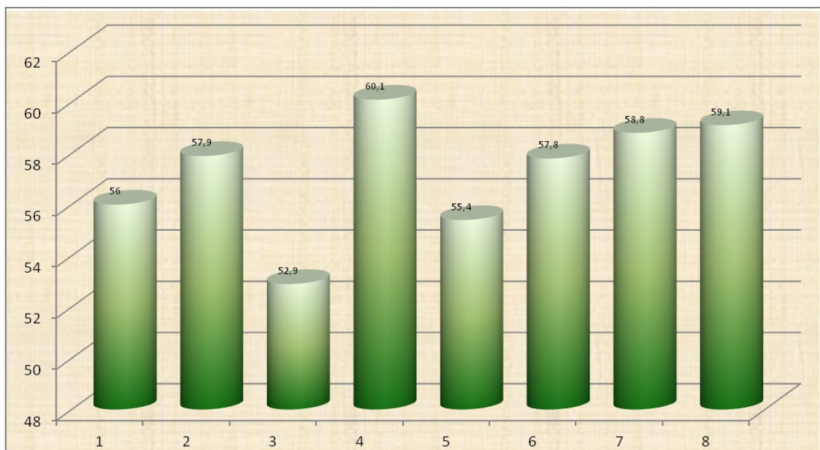
37 pav. Ekvivalentinio triukšmo pasiskirstymas matavimo vietose vakaro metu (18-22 val.). Ribinis dydis 60 dBA.
