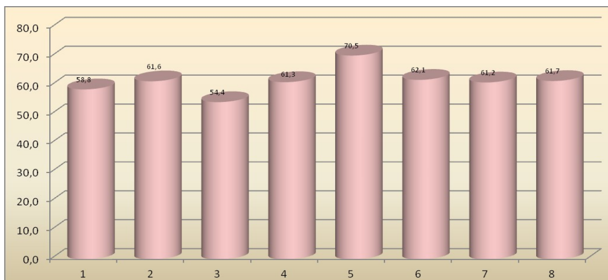
38 pav. Maksimalaus triukšmo pasiskirstymas matavimo vietose nakties metu (22-6 val.). Ribinis dydis 60 dBA.
